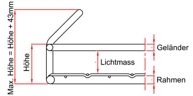
Schnitt A-A
