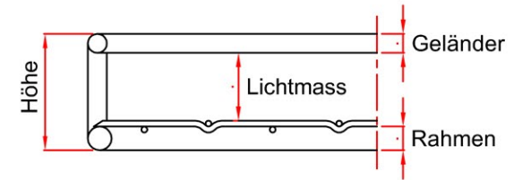
Schnitt A-A
