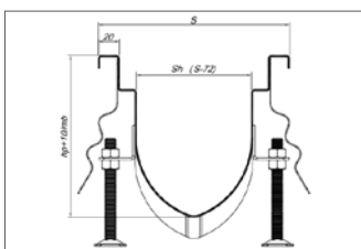
Smalle goot met halfronde bodem
