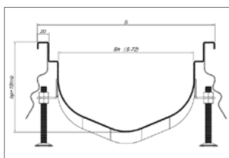
Brede goot met halfronde bodem
