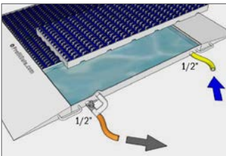
Aan- en afvoer 1/2" BI
